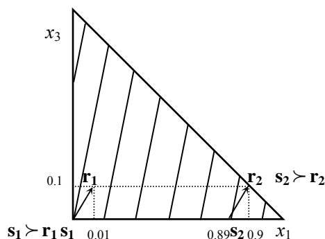
图 2 期望效用无差异曲线与 Allais 悖论
