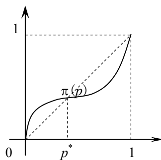
图 4 反“S”形概率权重函数
