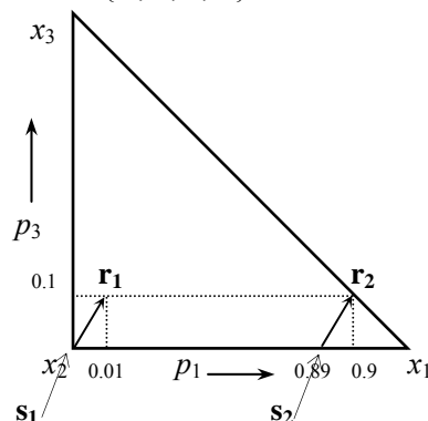
图 1 Machina 三角形中的 Allais 悖论
