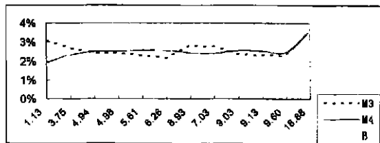
图 2 两种不同方法估计的债券价格结果比较
