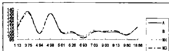
图 2 两种不同方法估计的债券价格结果比较
