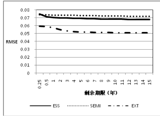
图 9 二阶矩样本外 RMSE
