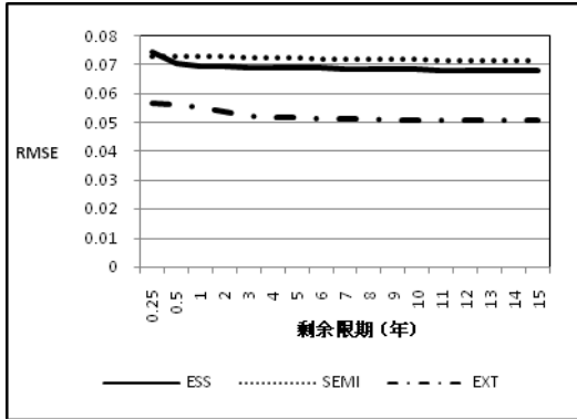
图 8 二阶矩样本内 RMSE
